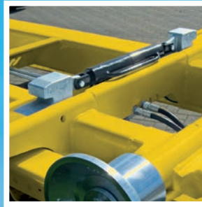
Combinatie-vergrendeling
